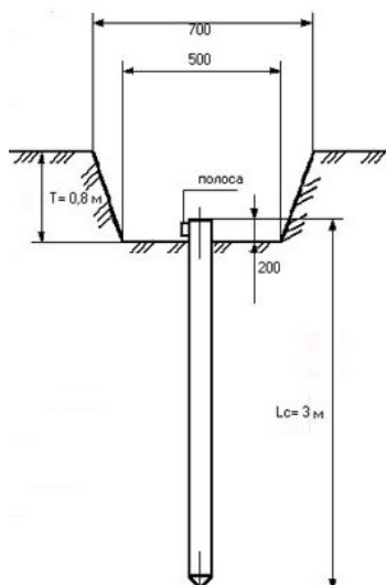
Электромонтаж очага заземления
