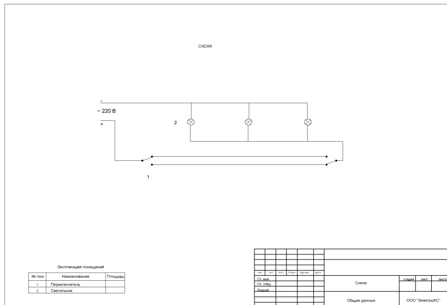
Схема расключения проходных выключателей
